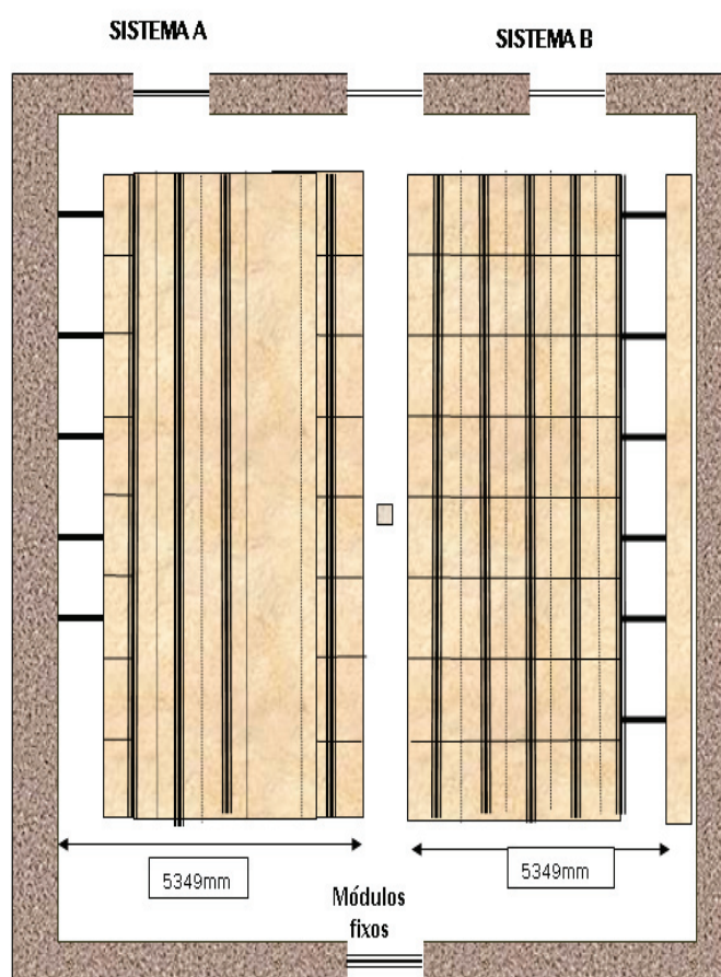
Figura 3 – Planta baixa de dois compactadores (verificar que a coluna disposta ao centro define seu posicionamento)
