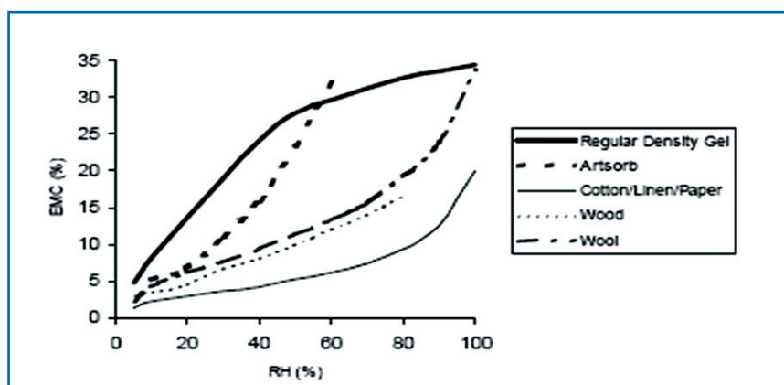
FIGURA 7 – Isotermas higroscópicas mostrando a variação de conteúdo de umidade em equilíbrio (EMC – Equilibrium Moisture Content) de duas sílicas-gel e de materiais orgânicos. Fonte: WEINTRAUB (2002), p. 2. Disponível em: < http://www.apsnyc.com/pdf/silica_gel_SW_2003.pdf > Acesso em: 15 nov. 2007.
